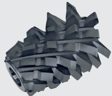
Schneckenrad-Wälzfräser zum Tangentialfräsen
