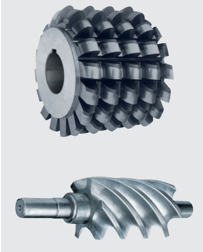
Nebenläufer Female rotor
