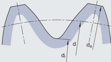
Werkstück Workpiece
