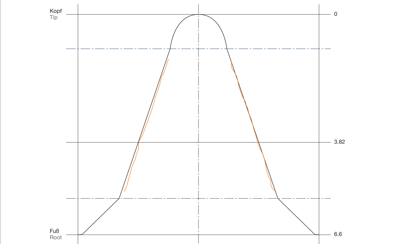
(12) Formabweichung der Schneidkante (12) Form deviation of the cutting edge
