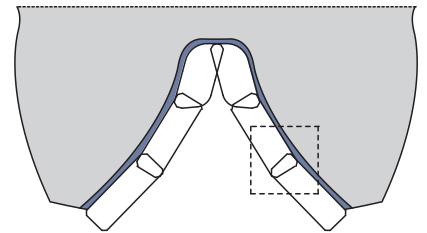
AV Schrappen angepasste Kontur Roughing of external gears with adapted contour
