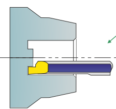
Обработка осевых канавок
